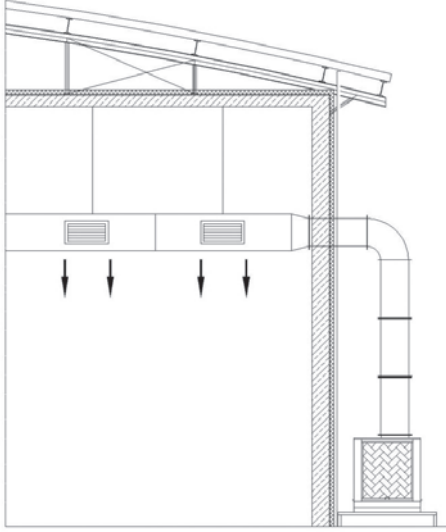
Üstten Üfleme Uygulaması FESKLİMA 35RCT - 30APT - 25APT
