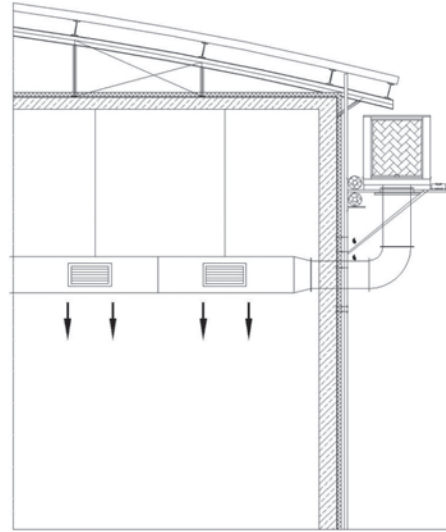
Alttan Üfleme Uygulaması FESKLİMA 35RCB - 20RPB - 16RPB - 10RPB - 30APB - 25APB
